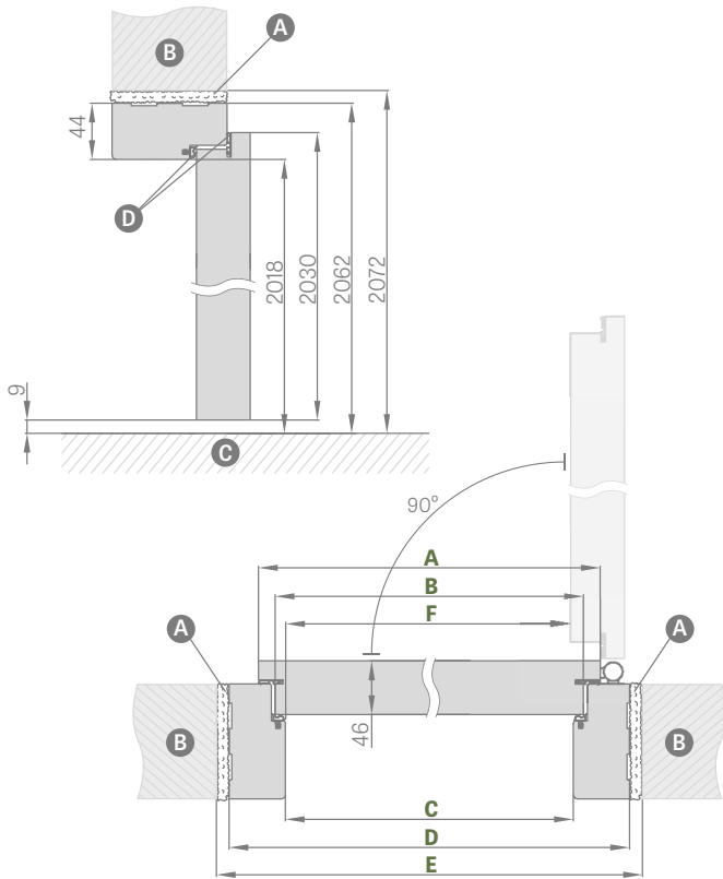
SCHÉMA DU DORMANT FIXE HERSE SET
