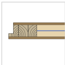
VANTAIL 46 mm renforcé par tôle acier
