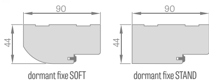
dormant fixe SOFT
