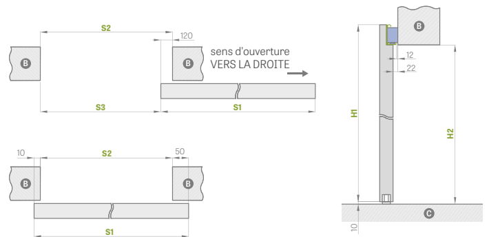
VANTAIL MAGIC, coloris CHÊNE PREMIUM, poignée ovale
