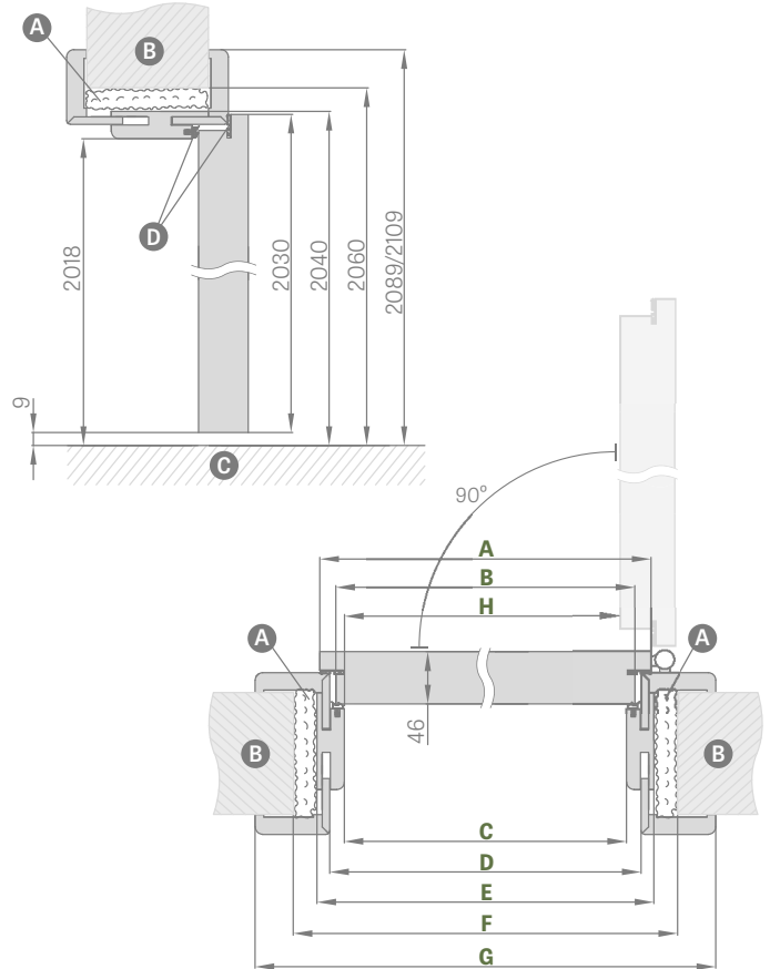
SCHÉMA DU DORMANT RÉGLABLE HERSE SET
